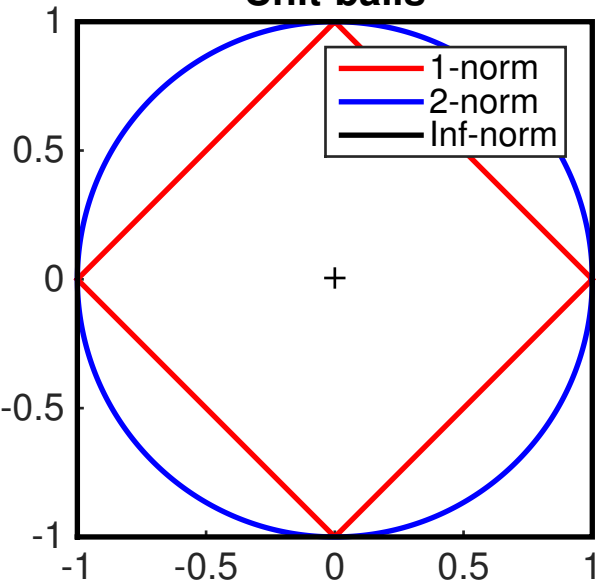
Unit-balls
